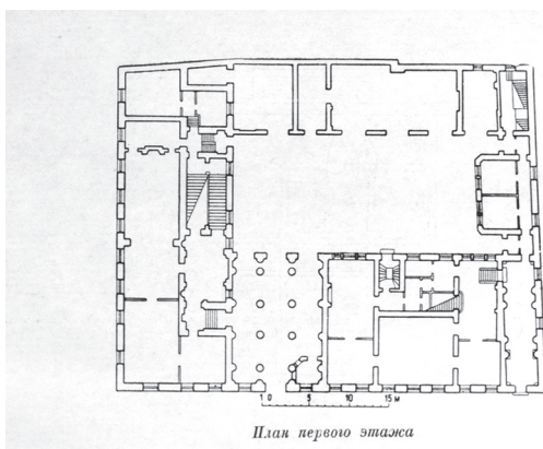
Рис. 9. Особняк Г.А. Тарасова в Москве. Арх. И.В. Жолтовский, 1909–1912. План 1-го этажа.
